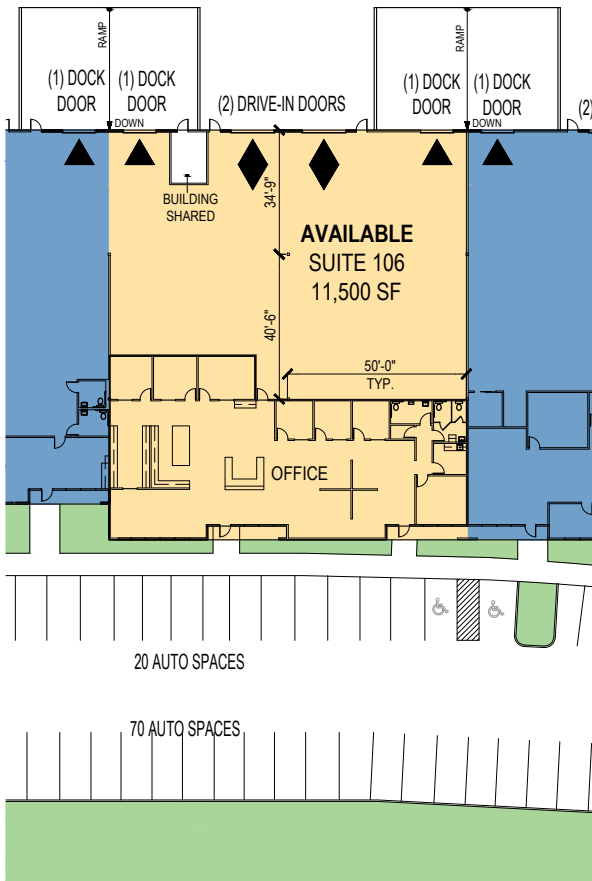
SUITE 106 PLAN
